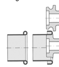
Zulegwalzen ZB
