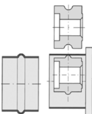
Sickenwalzen S
